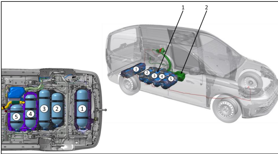
Figure 1 : schéma de principe, vue des réservoirs de gaz et d'essence
