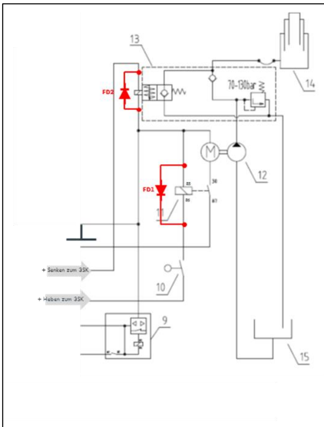
Schéma de principe : exemple de circuit de commande de benne basculante
