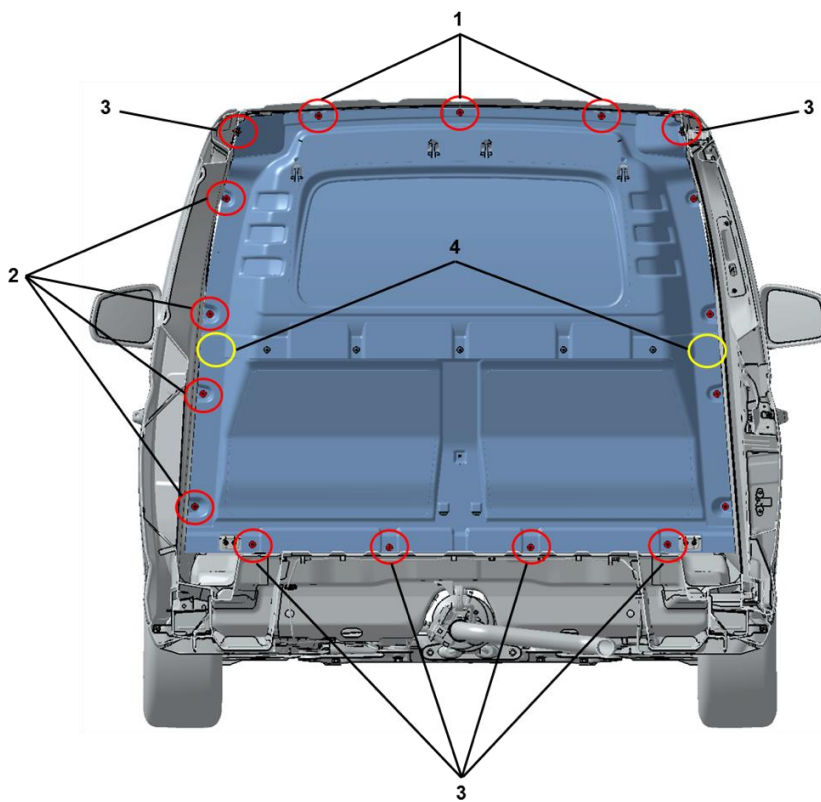
Fig. 2 : points de fixation pour la cloison de série (coupe A-A)
