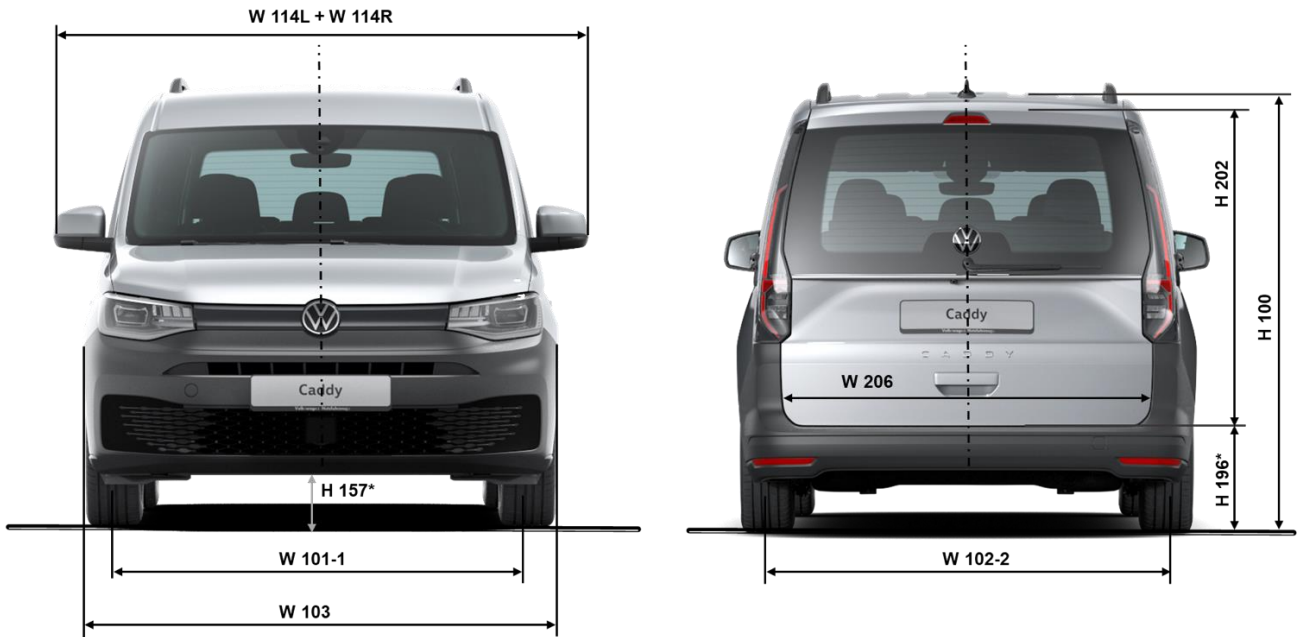
Fig. 2 : cotes du Caddy/Caddy Maxi, vue de devant et de derrière (conformément à la norme DIN70020, partie 1)
