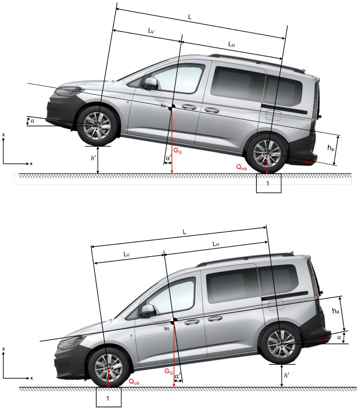
Fig. 2 : détermination de la position du centre de gravité global du véhicule dans le sens z
