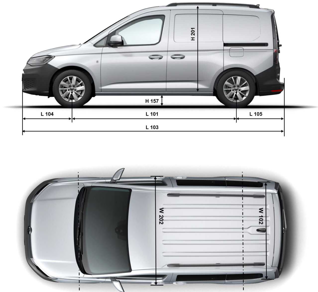
Fig. 1 : cotes du Caddy (selon la norme DIN70020, partie 1)
