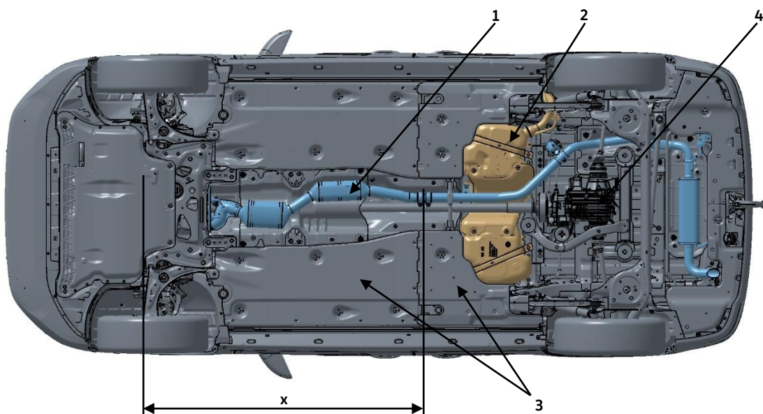
Fig. 1: impianto di scarico 4x4 (integrale), passo corto (fig.: trazione 4x4, 90KW TDI)
