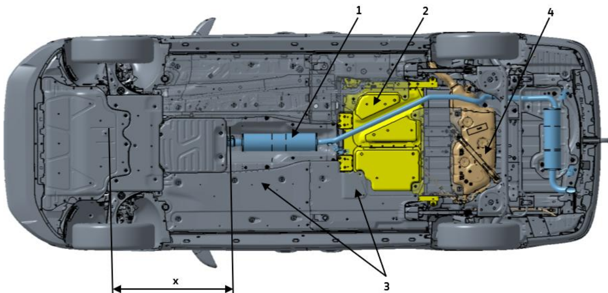
Fig. 2: impianto di scarico PHEV, passo lungo (figura trazione 4x2, 85KW TSI)
