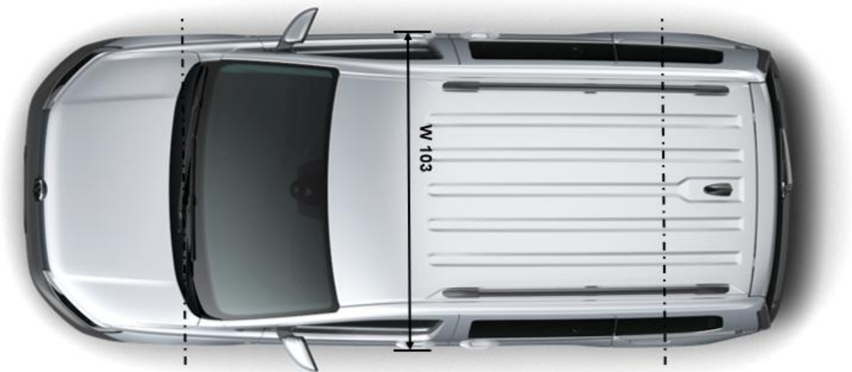
Fig. 2: Dimensioni Caddy (secondo la norma DIN70020, parte I)
