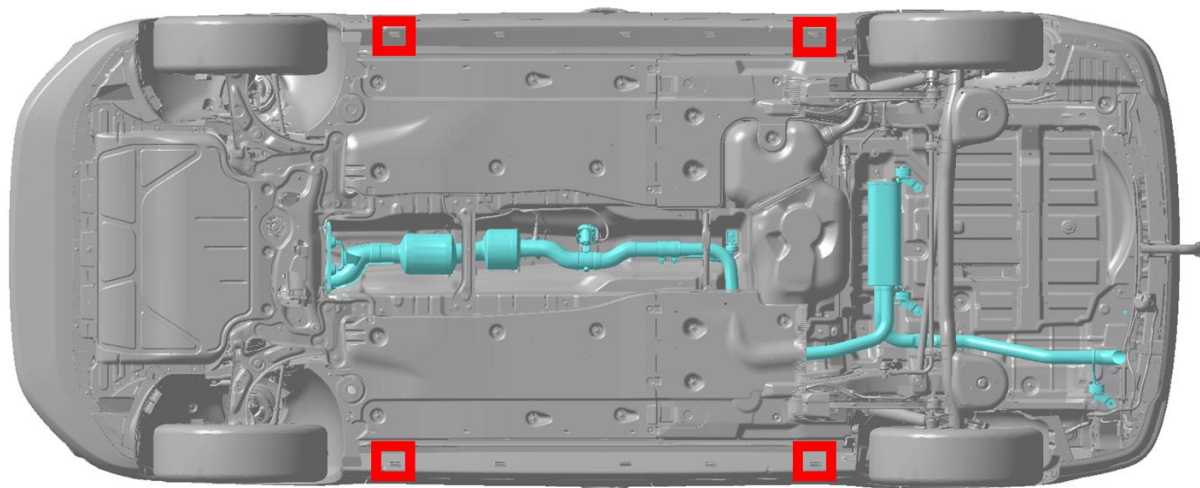
Fig. 1: punti di sollevamento per il cric (esempio)
