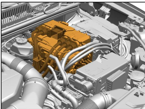
Fig. 2: sistema elettronico comandi ed erogazione per trazione elettrica
