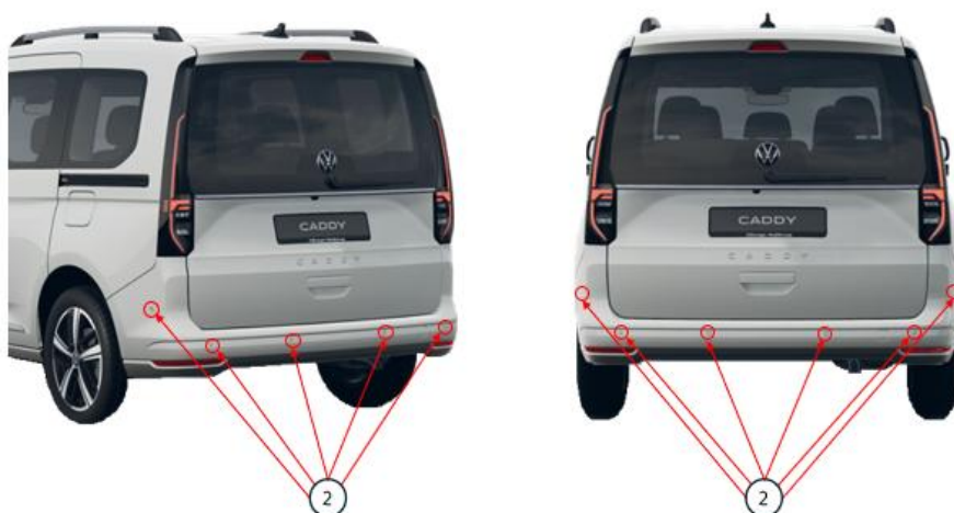
Fig. 2: posizione dei sensori PDC dietro
