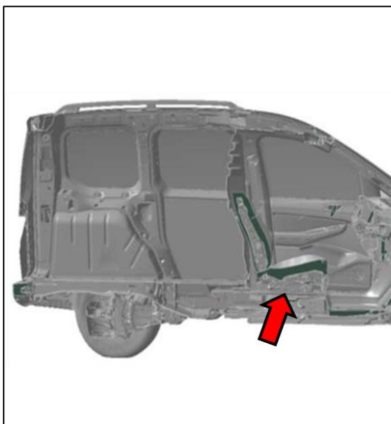
Fig. 1: posizione del punto di accoppiamento della predisposizione
