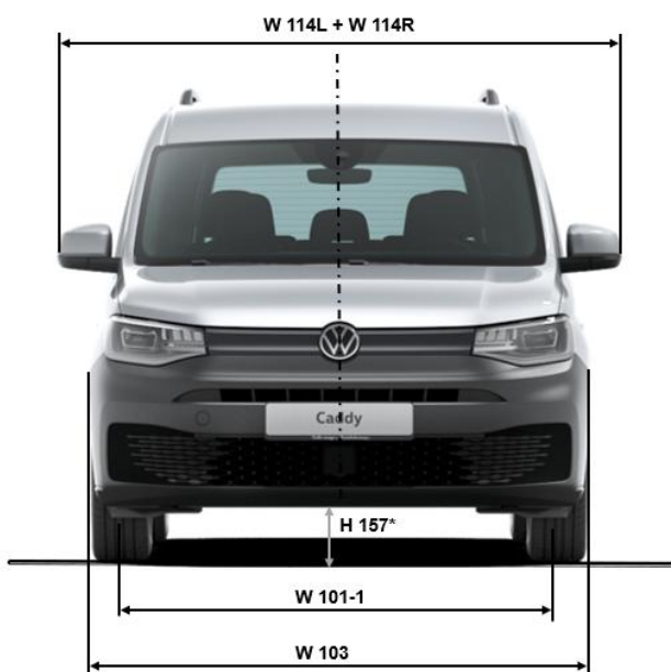
Fig. 3: Dimensioni Caddy o Caddy Maxi, vista anteriore (conforme a DIN70020, T1)
