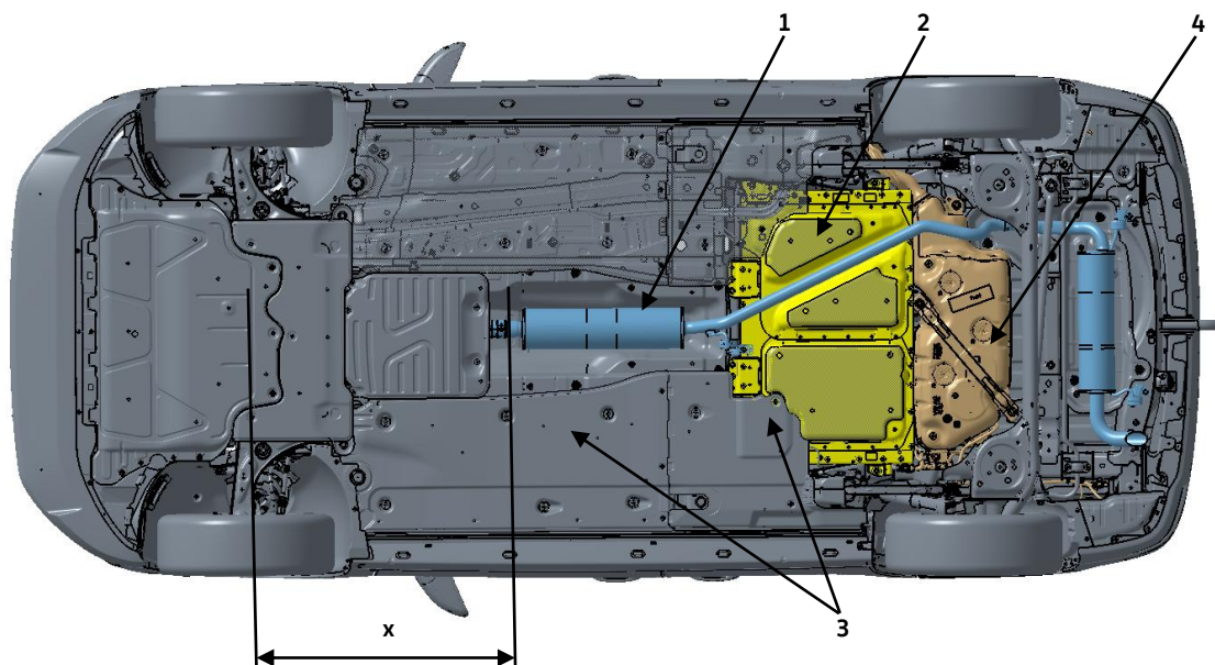
Fig. 1: impianto di scarico PHEV, passo corto (fig.: trazione 4x2, 85KW TSI)
