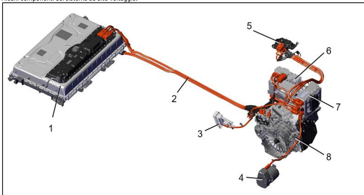
Fig. 1: i componenti più importanti della trazione elettrica
