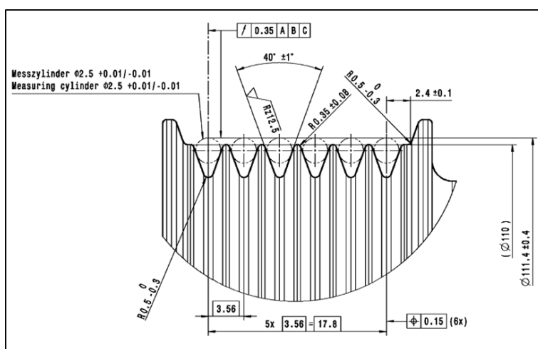
Fig. 1: Particolare U - puleggia del compressore del climatizzatore (esempio Denso 7SAS17)
