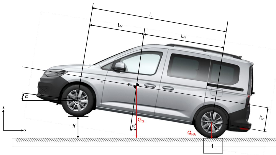
Fig. 1: Calcolo della posizione del baricentro complessivo del veicolo in direzione z
