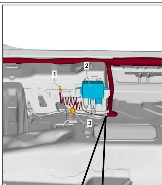
Fig. 2: lato interno del telaio del sedile sinistro
