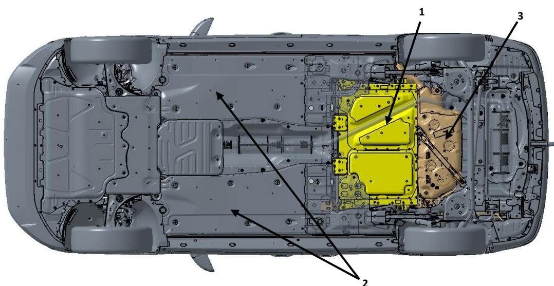
Fig. 2: vista dal basso, versione a passo corto: posizione della batteria ad alto voltaggio
