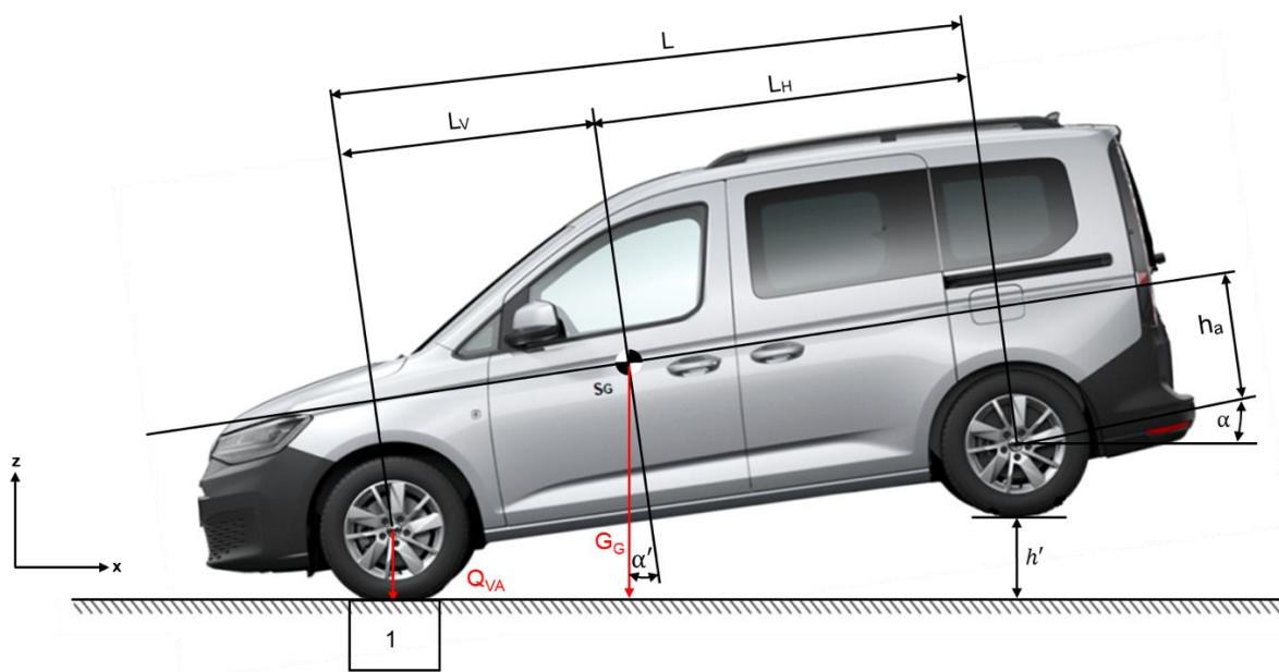
Fig. 2: Calcolo della posizione del baricentro complessivo del veicolo in direzione z
