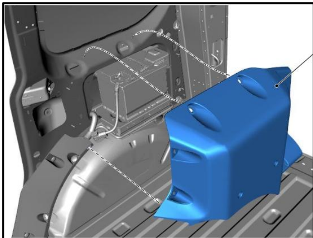
Fig. 1: batteria di avviamento con copertura nella zona posteriore destra del vano di carico, sopra il passaruota
