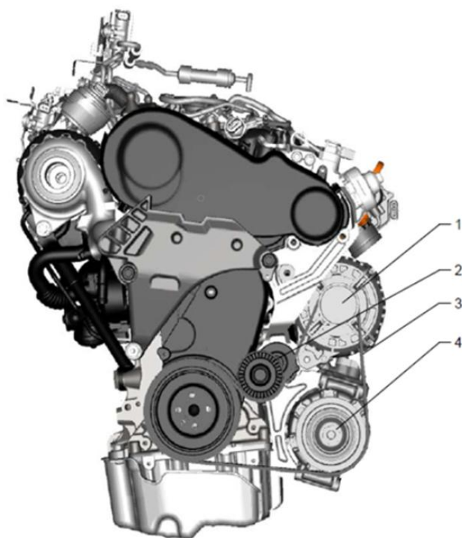
Fig. 2: rappresentazione esemplificativa dell'azionamento con cinghia poli-V
