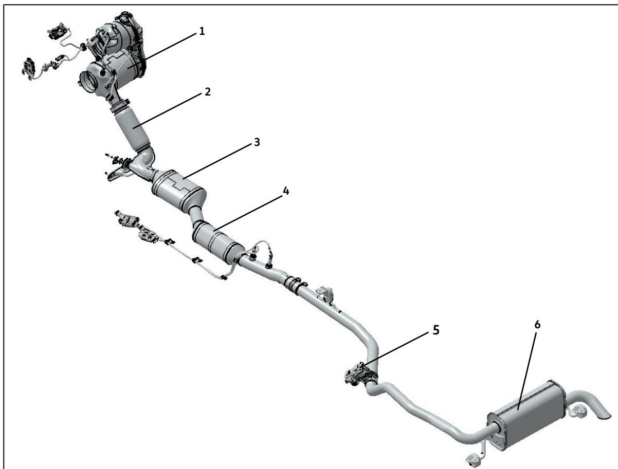
Fig. 3: depurazione dei gas di scarico con sistema SCR
