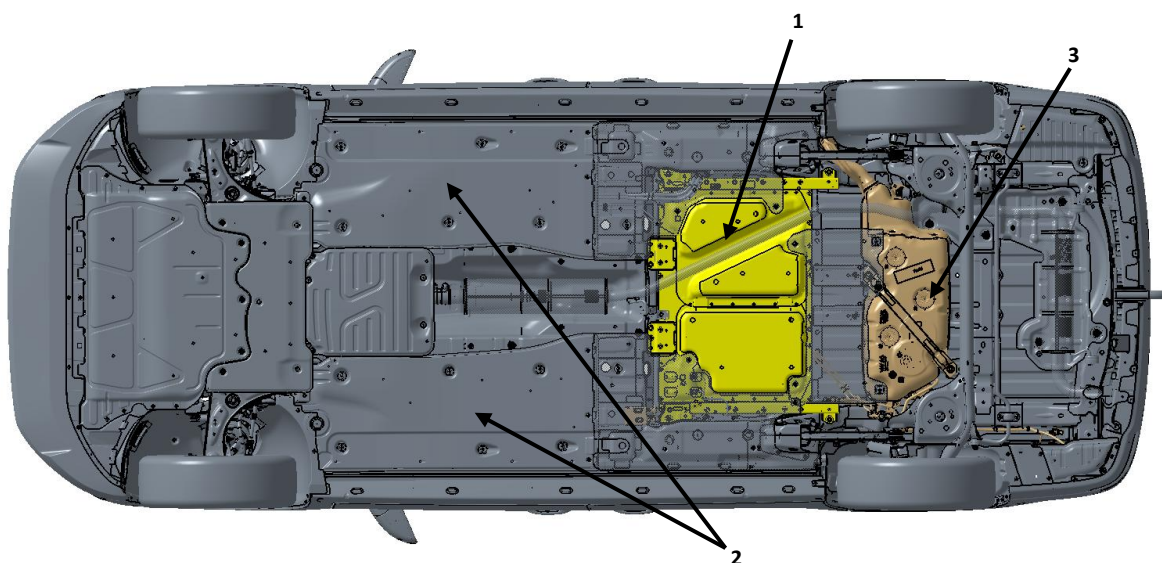
Fig. 1: vista dal basso, versione a passo lungo: posizione della batteria ad alto voltaggio
