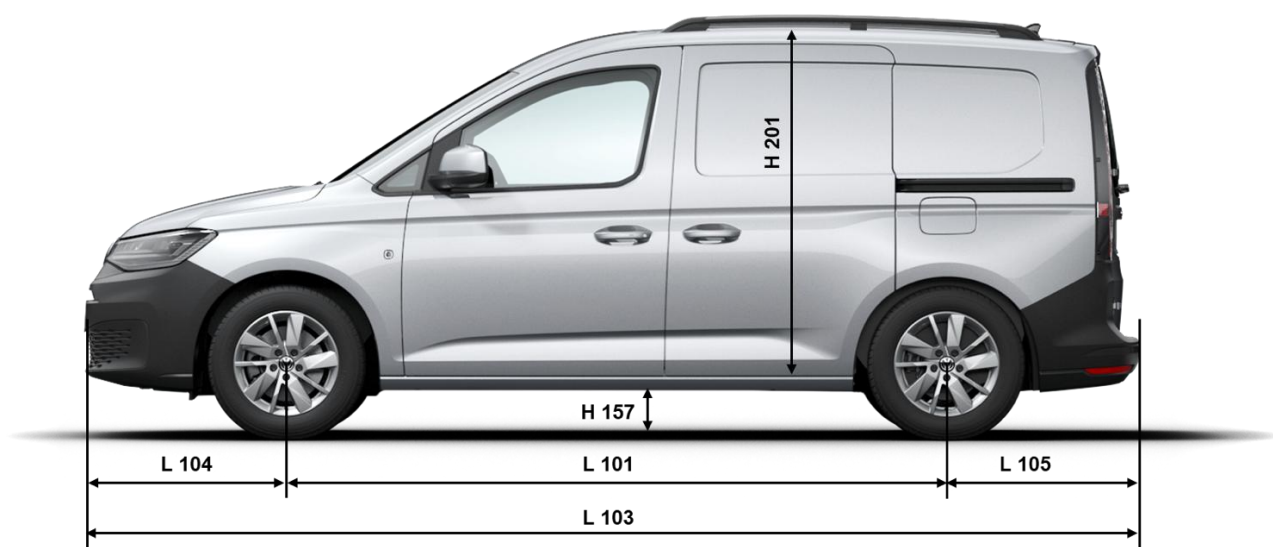
Fig. 1: Dimensioni Caddy (secondo la norma DIN70020, parte I)
