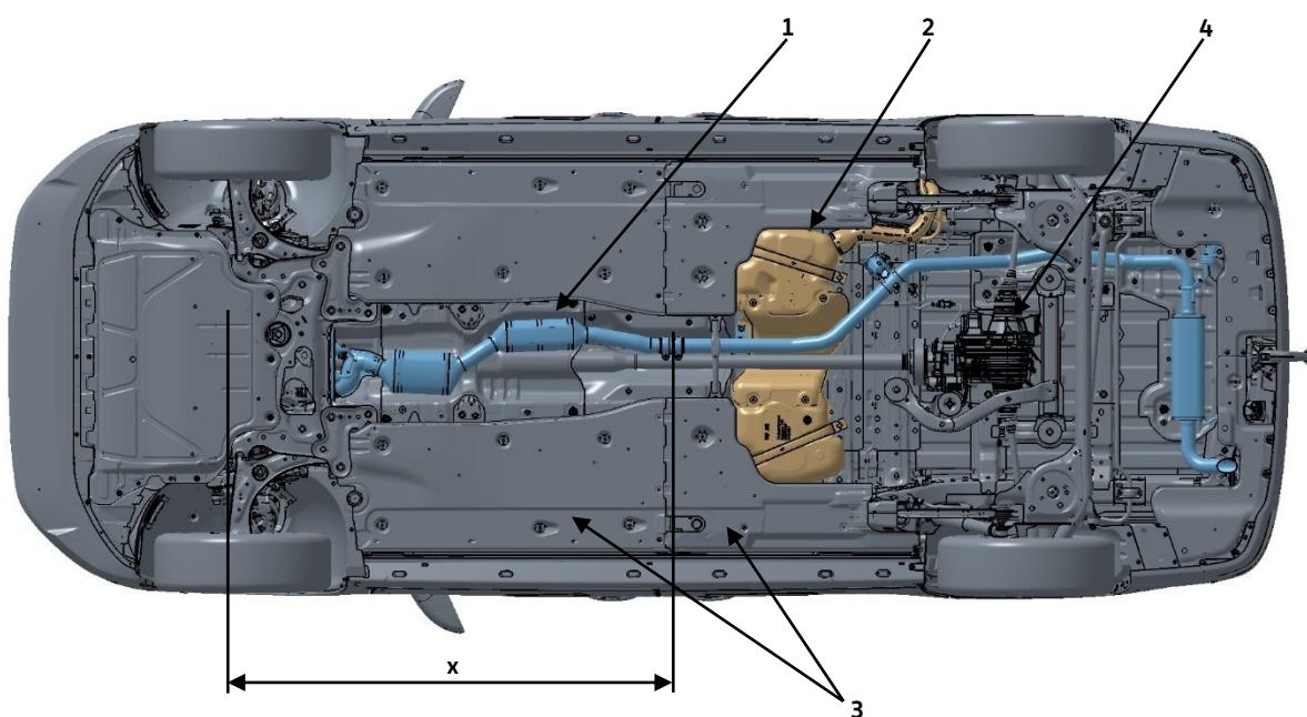
Fig. 2: impianto di scarico 4x4 (integrale), passo lungo (fig.: trazione 4x4, 90KW TDI)
