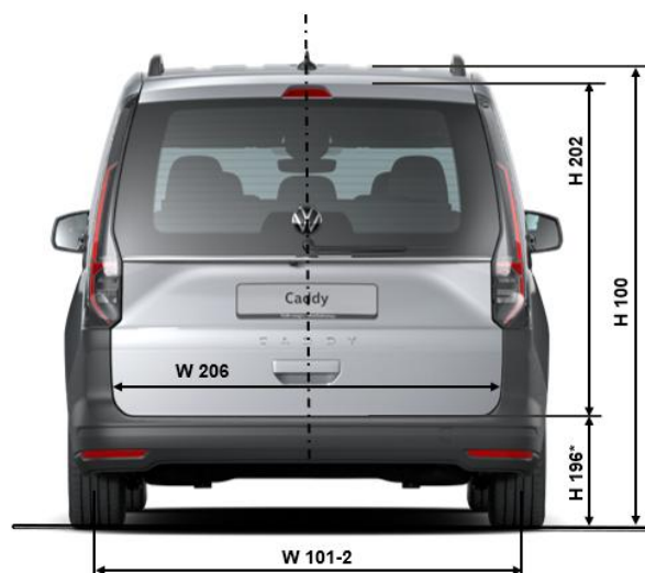
Fig. 4: Dimensioni Caddy o Caddy Maxi, vista posteriore (conforme a DIN70020, T1)
