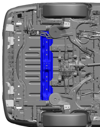
Fig. 2 : traverse sur la version ICE AWD
