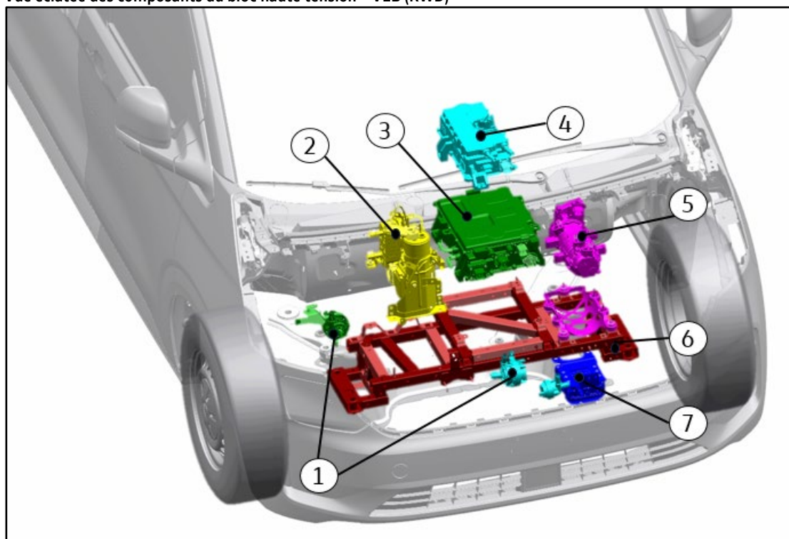
Vue éclatée des composants du bloc haute tension – VEB (RWD)
