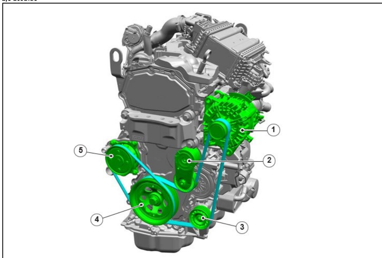
Fig. 1 : Moteur sans AC
