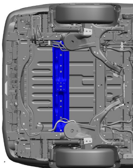
Fig. 3 : traverse sur la version ICE FWD avec roue de secours ou roue d'urgence
