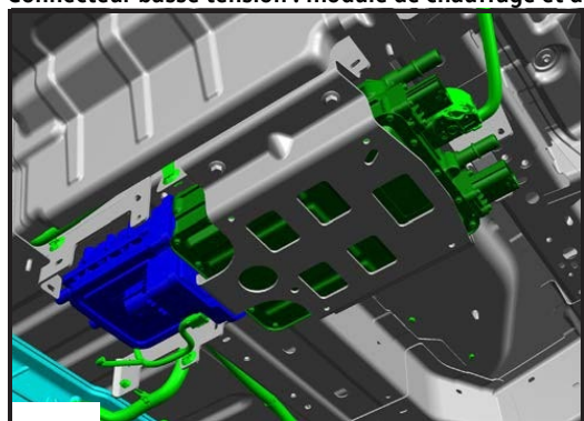
Connecteur basse tension : module de chauffage et de charge – VHR
