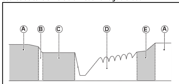
Courbe de tension lors d'un redémarrage à chaud
