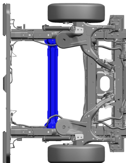
Fig. 6 : traverse sur la version ICE double cabine FWD sans roue de secours
