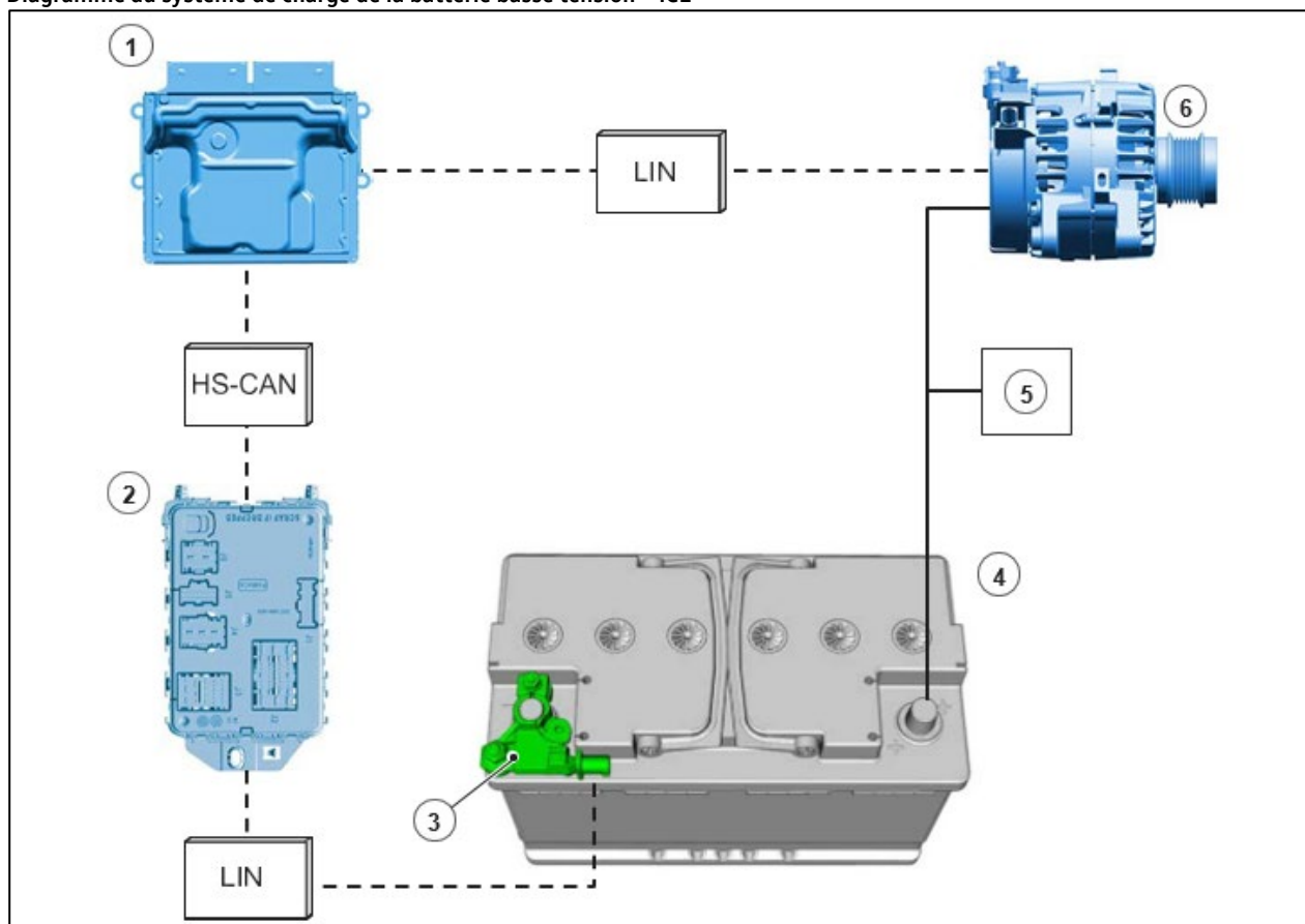
Diagramme du système de charge de la batterie basse tension – ICE
