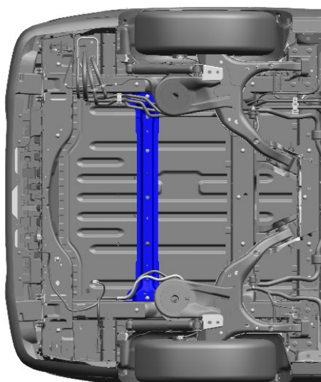
Fig. 1 : traverse sur la version ICE FWD sans roue de secours
