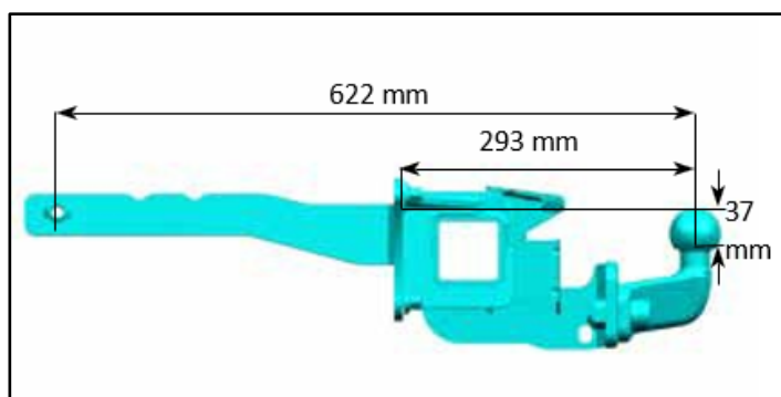
Fig. 2 : dispositif d'attelage vissé
