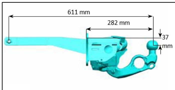
Fig. 1 : dispositif d'attelage escamotable
