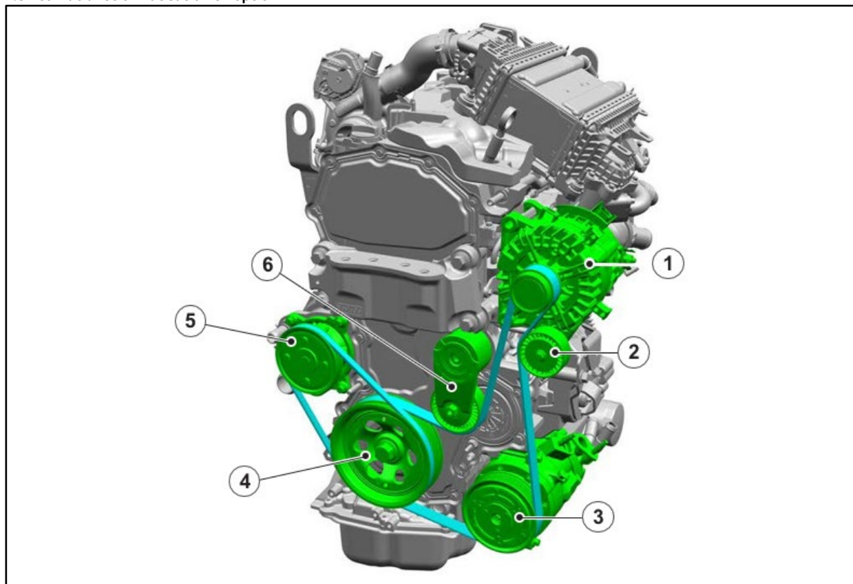
Fig. 2 : Moteur avec AC en option
