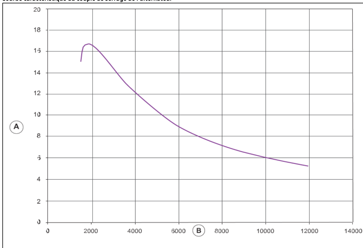
Courbe caractéristique du couple de serrage de l'alternateur
