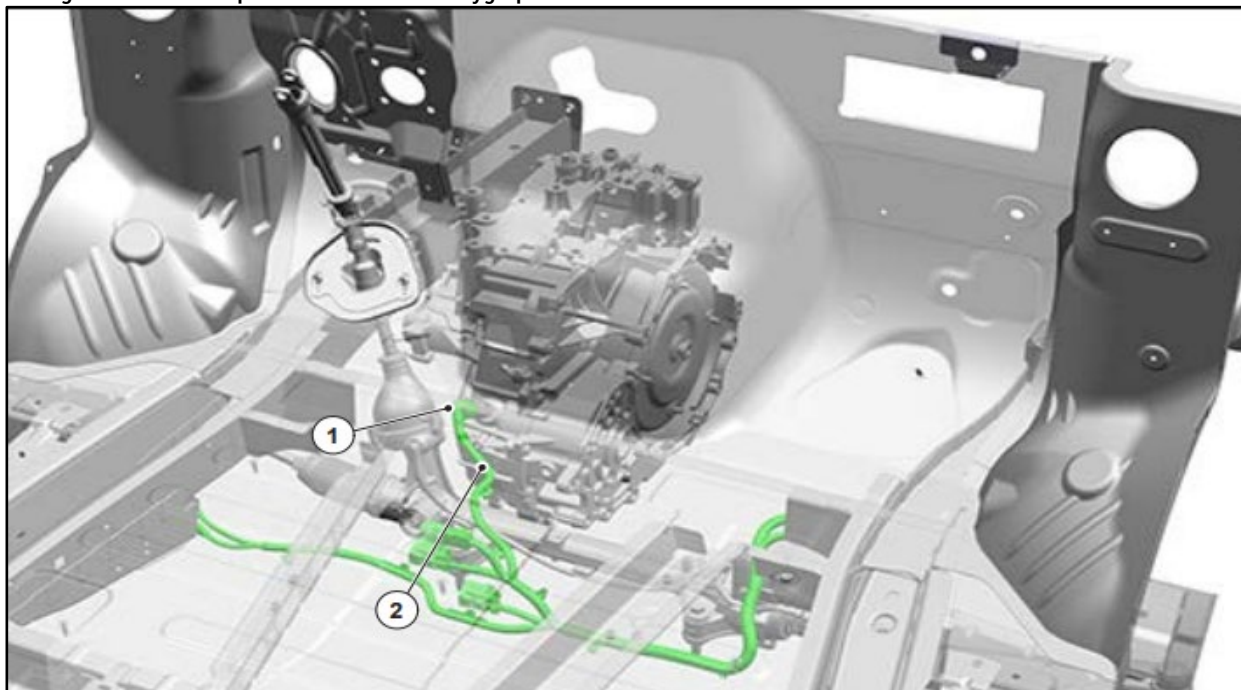
Fig. 1 : Passage des câbles – Capteur de vitesse du tachygraphe
