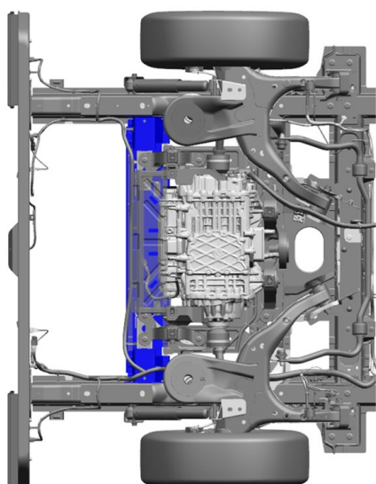
Fig. 9 : traverse sur la variante VEB double cabine RWD
