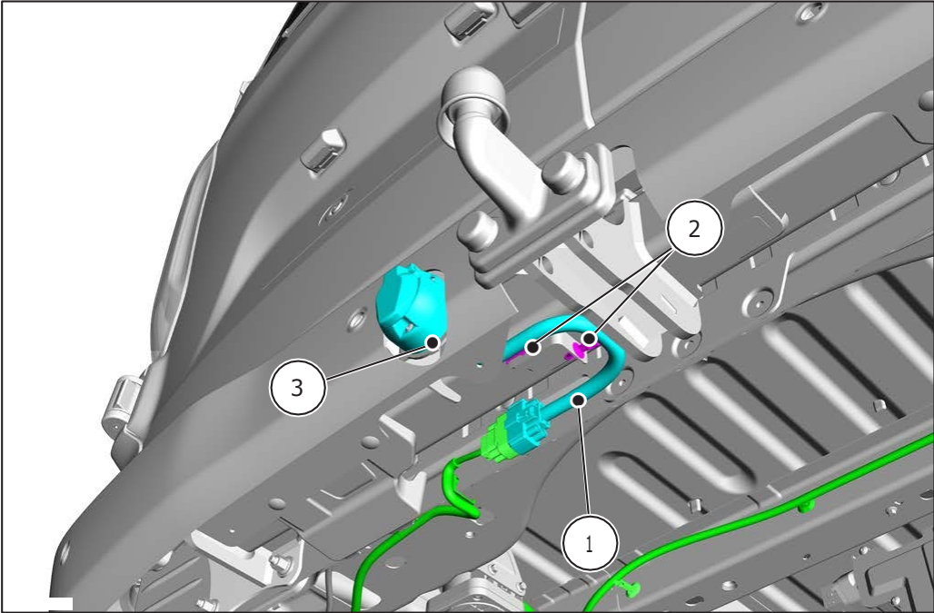
Kit de câblage, système électrique pour dispositif d'attelage (numéro PR 1M5)
