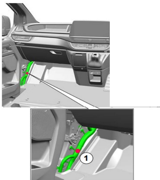
Figure : véhicule représenté avec conduite à droite, même position de la boucle de câble pour conduite à gauche
