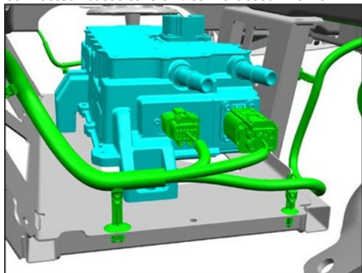
Connecteur basse tension : convertisseur DC AC – VHR
