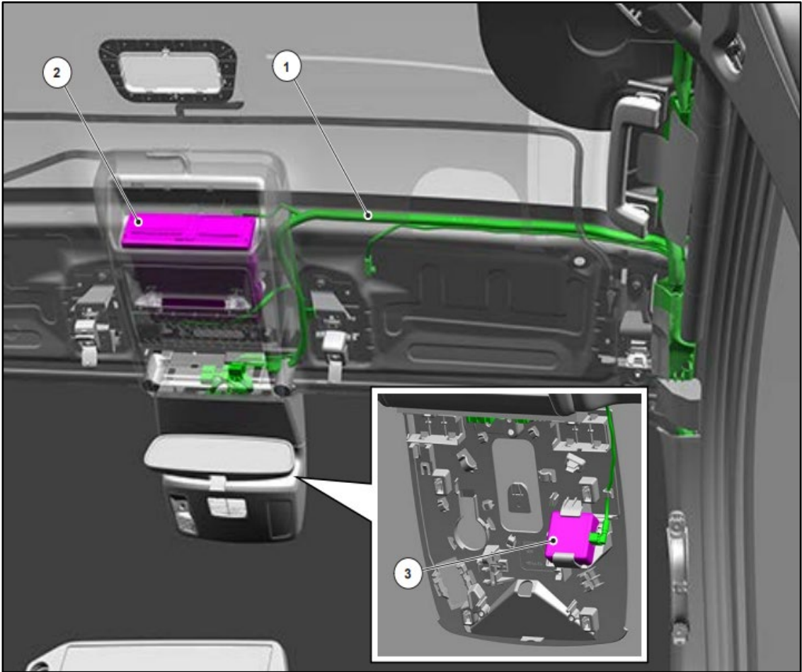
Fig. 2 : Câblage électrique – Tachygraphe et module DSRC
