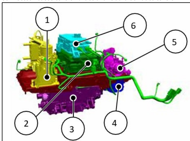
Connecteur basse tension : face avant du bloc haute tension – VEB (AWD)
