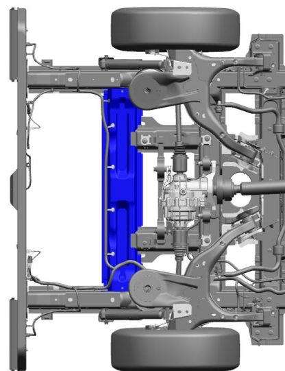
Fig. 7 : traverse sur la version ICE double cabine AWD
