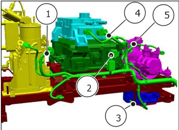
Connecteur basse tension : face avant du bloc haute tension – VEB (RWD)
