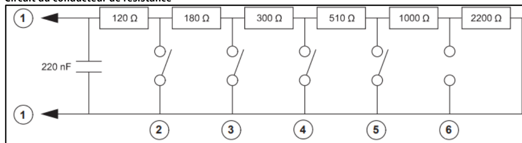
Circuit du conducteur de résistance
