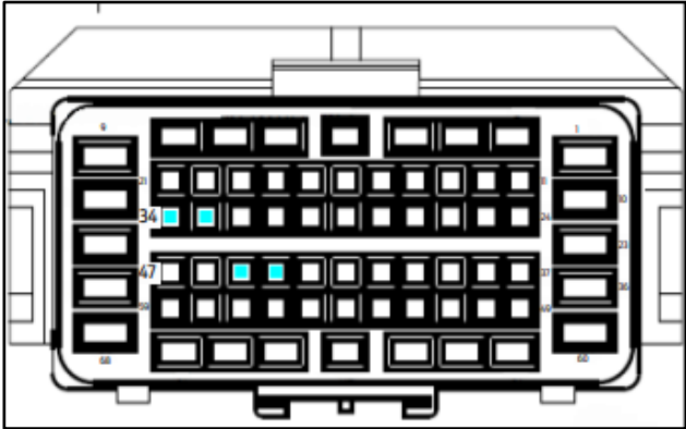
Connecteurs pour les haut-parleurs arrière
