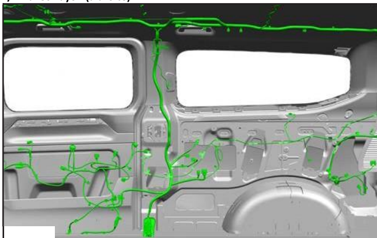
L2/H1 avec hayon (à droite)
