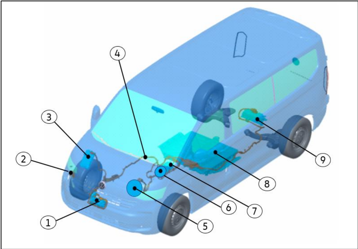
Vue d'ensemble du système haute tension – VHR
