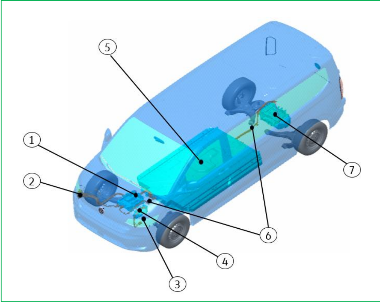
Vue d'ensemble du système haute tension – VEB
