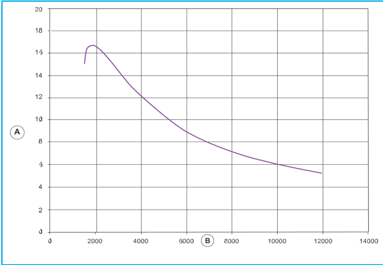
Courbe caractéristique du couple de serrage de l'alternateur
