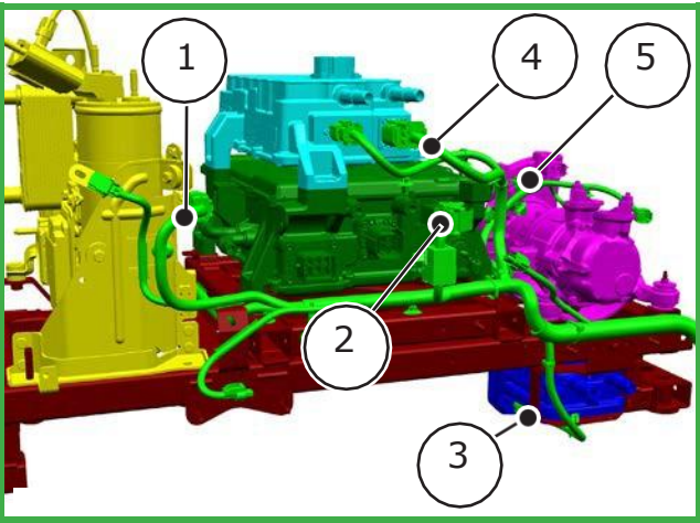
Connecteur basse tension : face avant du bloc haute tension – VEB
