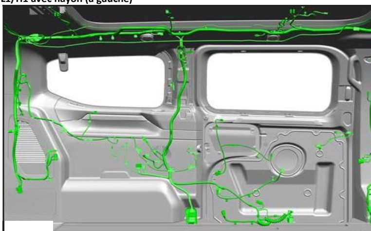
L1/H1 avec hayon (à gauche)
