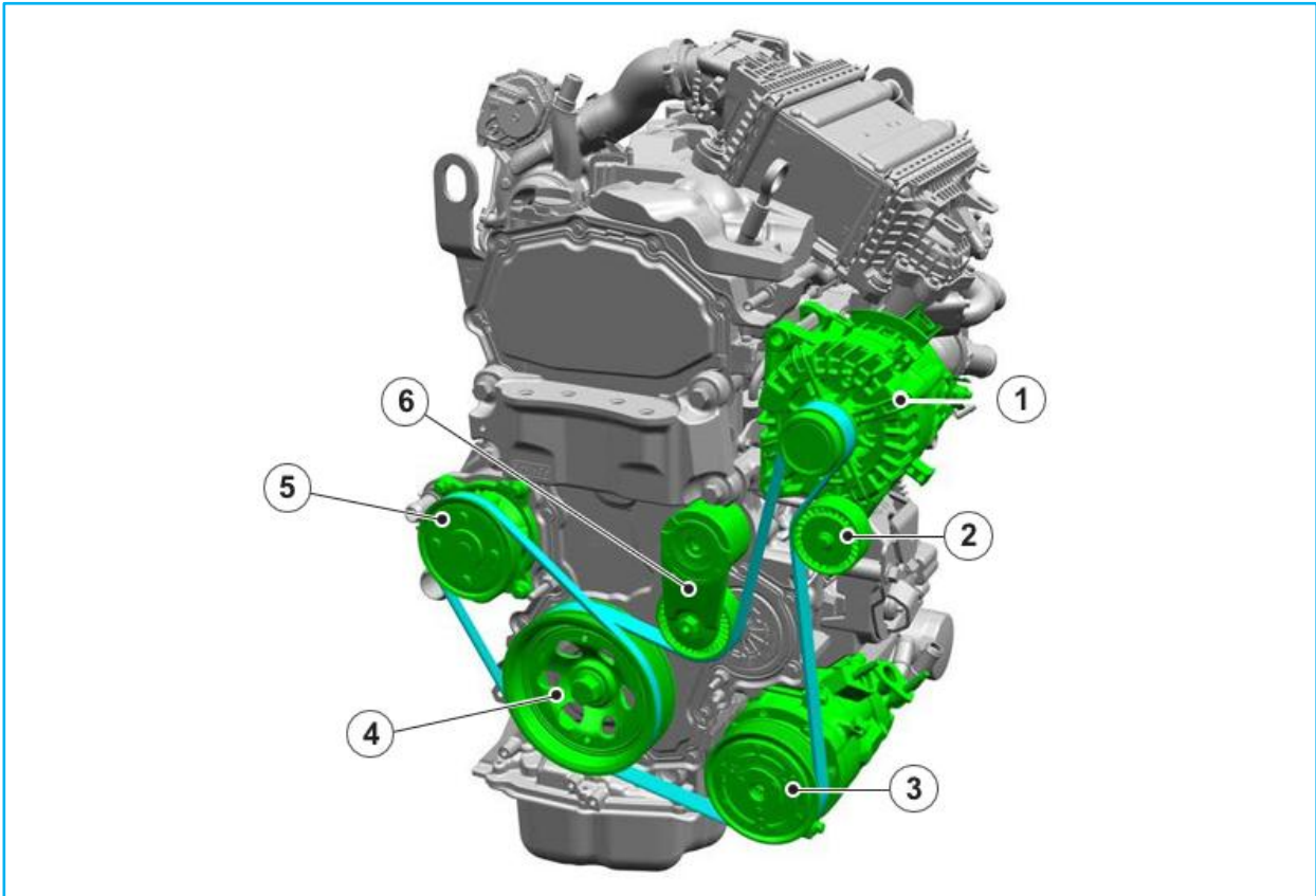
Fig. 2 : Moteur avec AC en option
